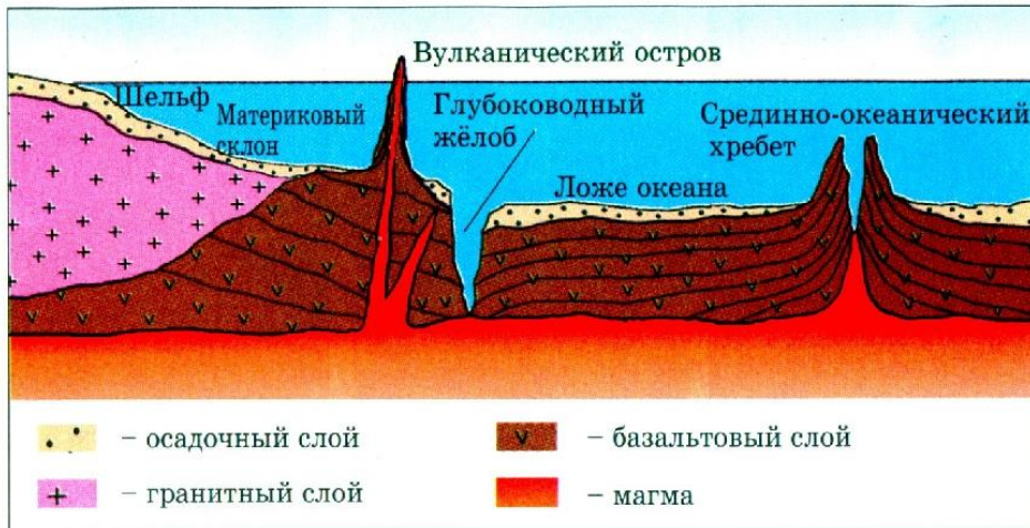
Рельеф дна океана
